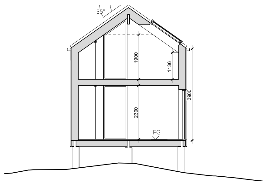
SEKTION A-A
