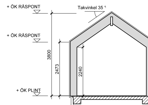
SEKTION
