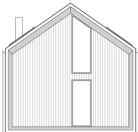
FASAD MOT NORDÖST
