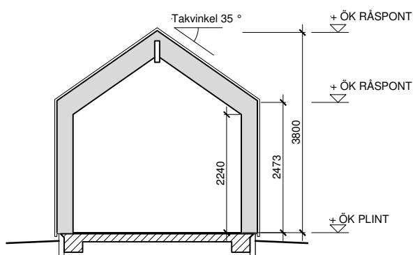
SEKTION
