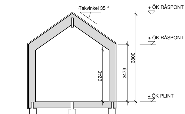
SEKTION
