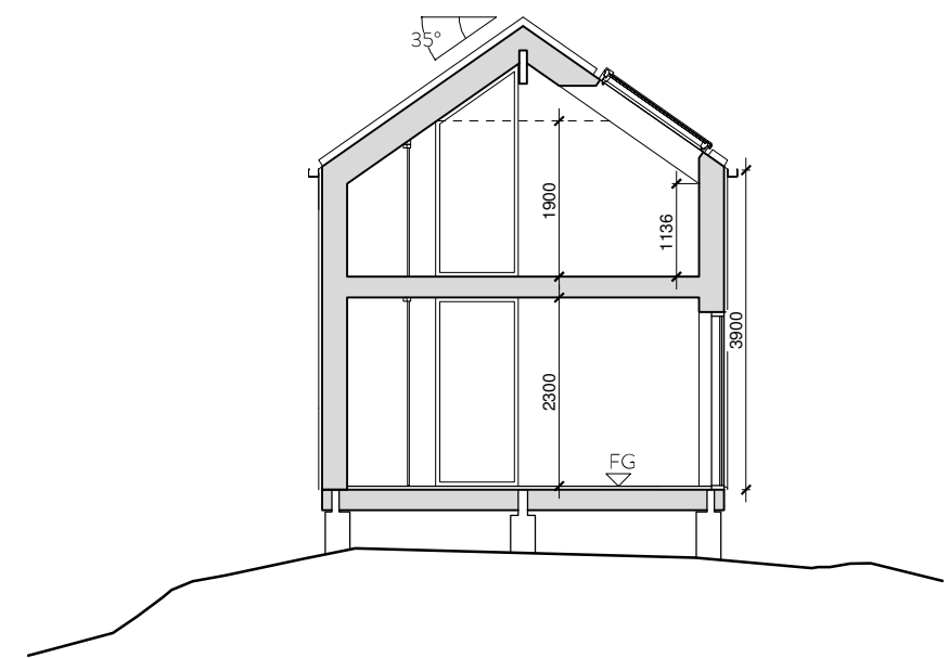
SEKTION A-A
